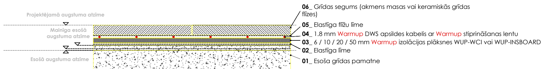
WARMUP DWS APSILDES KABELIS AR STIPRINĀŠANAS LENTU UZ BETONA PAMATNES
