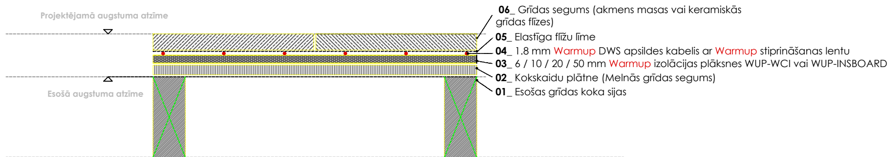
WARMUP DWS APSILDES KABELIS AR STIPRINĀŠANAS LENTU UZ KOKA KONSTRUKCIJU PAMATNES
